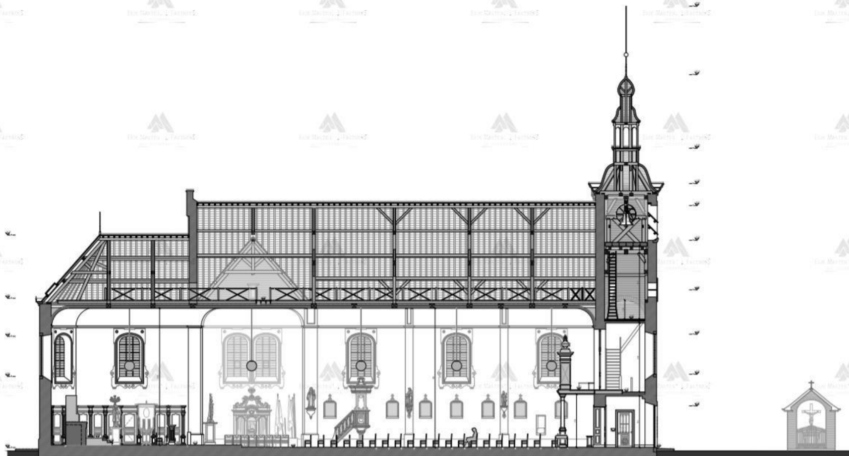
snede A-A bestaande toestand - schaal 1:150
