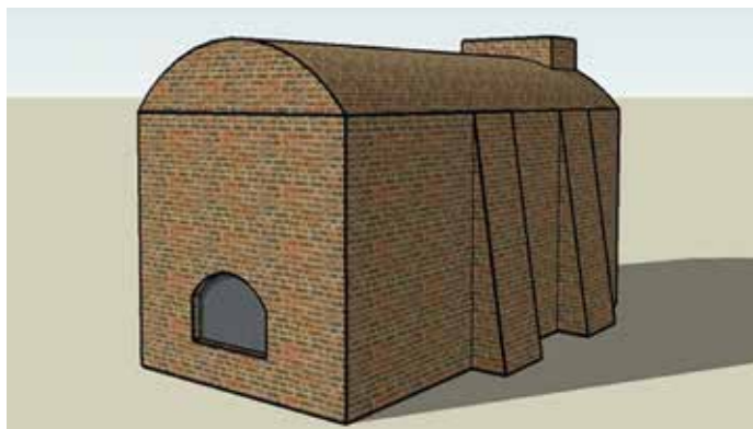
Een reconstructie van de pannenoven zoals die door de Schulense pannenbakkers werd gebruikt. Vooraan de deur waarlangs werd gestookt. De opening waarlangs de oven werd geladen bevindt zich aan de achterkant. (Foto: Patrick Boucneau)
